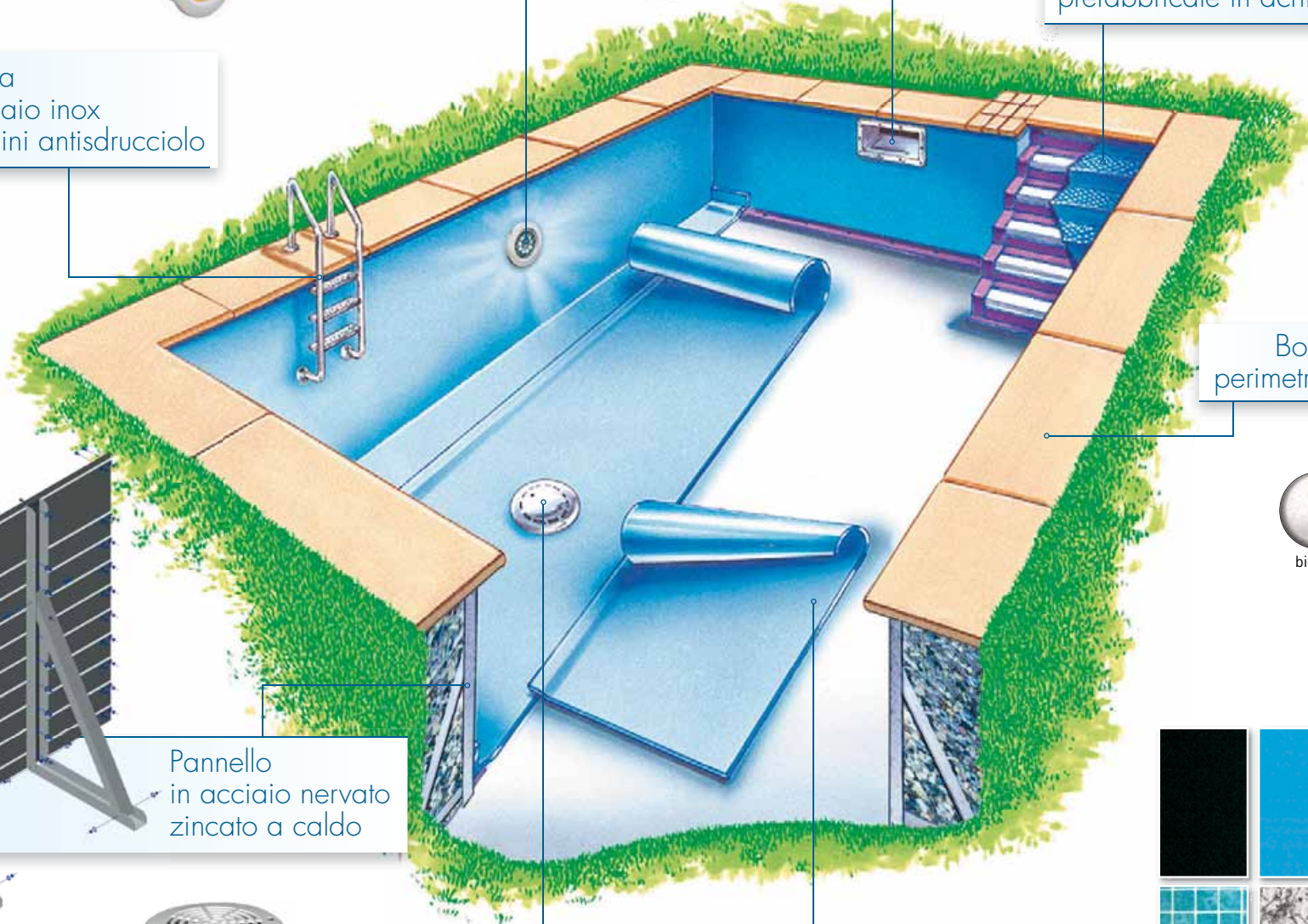
Scalinate in opera da rivestire o scalinate prefabbricate in acrilico
